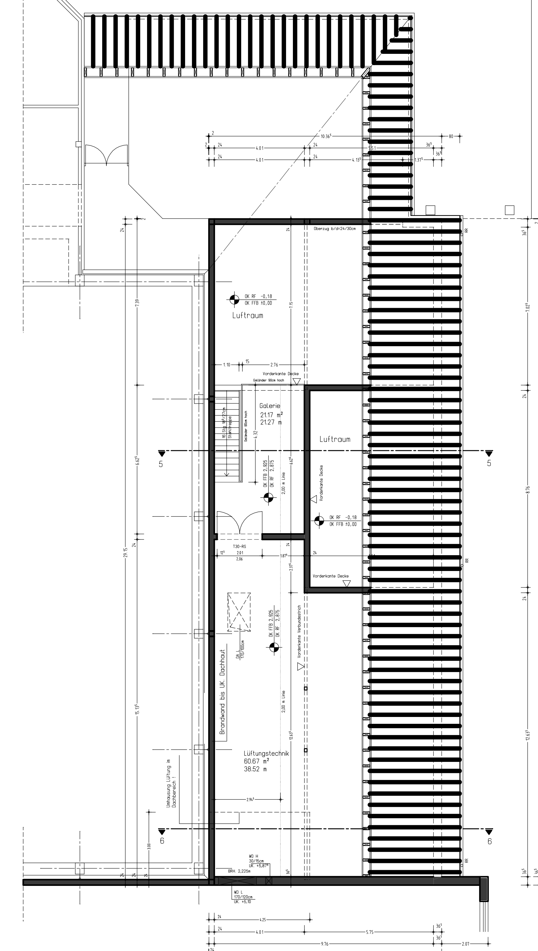
Grundriss Dachboden Hausmeister, Lüftungszentrale
